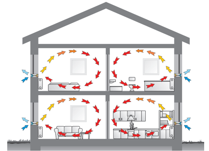
Dezentrale Lüftungsanlage
