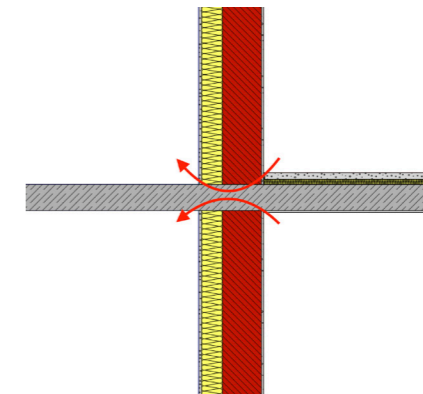
b.) Konstruktive Wärmebrücke
