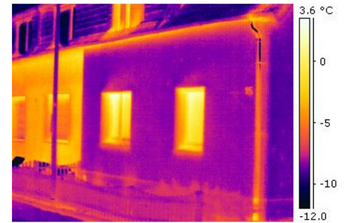
Thermografie eines gedämmten und nicht gedämmten Hauses. Allerdings wurde die Fensterlaibung nicht gedämmt.
