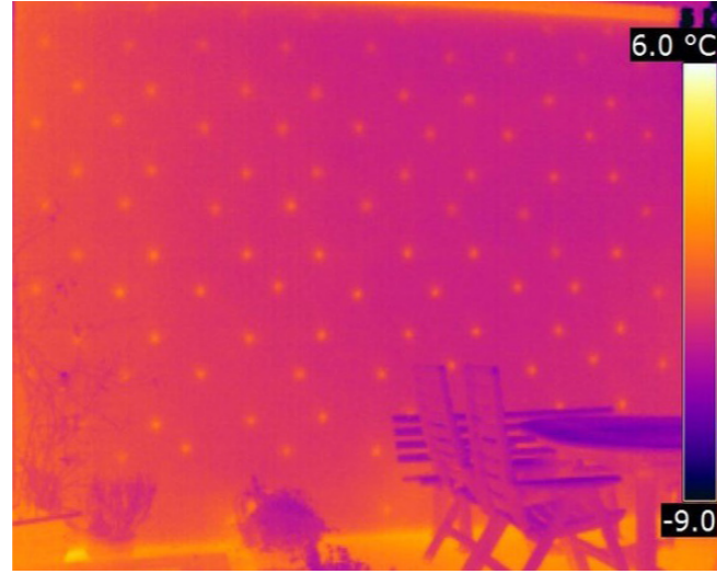
Dalmatiner-Effekt durch die Dübel beim Wärmedämmverbundsystem (WDVS)
