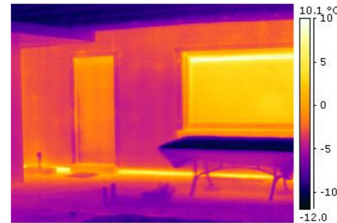
Thermografie eines nicht gedämmten Sockelanschlusses
