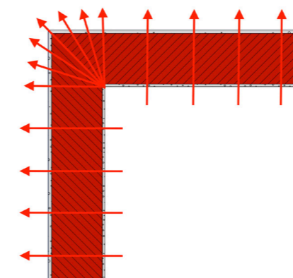
a.) Geometrische Wärmebrücke
