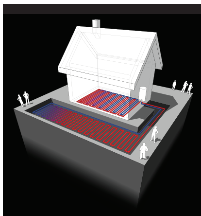
Sole-/Wasser-Wärmepumpe
