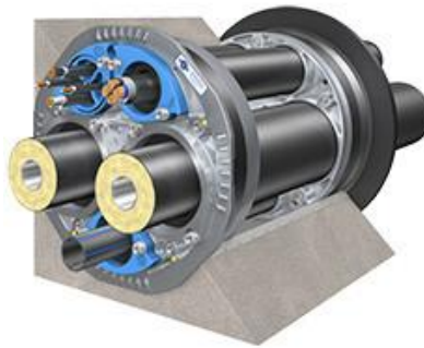
Abb. 6: Beispiel einer Mehrsparten-Hauseinführung (Quelle: Doyma)
